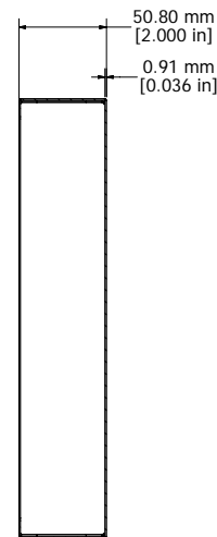
SECTION JJ-JJ
