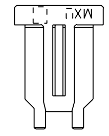
2極品形状 VIEW OF 2 CKT.
