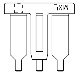
3極品形状 VIEW OF 3 CKT.
